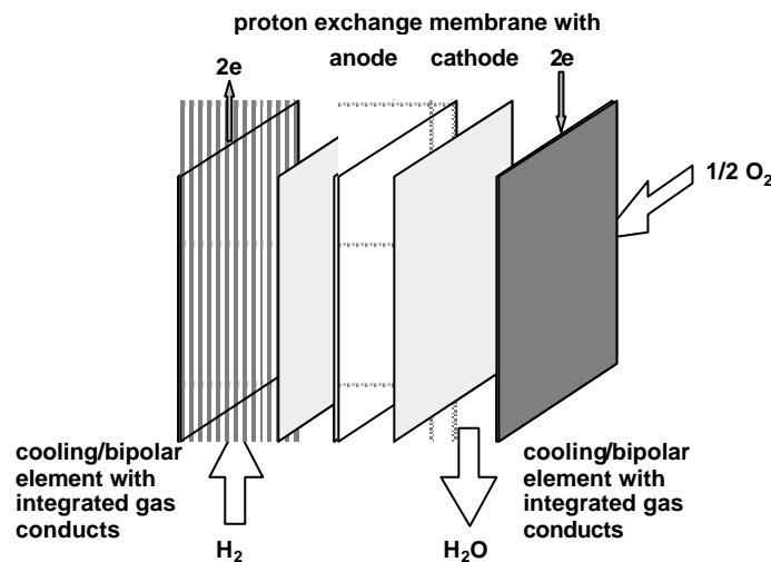
Aufbau einer Wasserstoff-Sauerstoff-Brennstoffzelle
