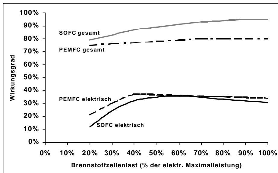
Kennlinien für SOFC -Zellen mit 1 \text{ kW}_{el} und eine PEMFC -Zelle mit 4,5 \text{ kW}_{el} Leistung bei Erdgasbetrieb (Quelle: Bokemper 2001) 4
