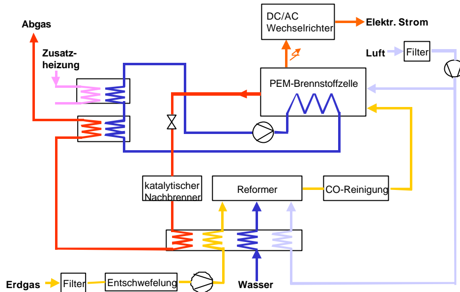
Denkbares Schaltungssystem eines PEMFC-Heizsystems mit Erdgasreformer
