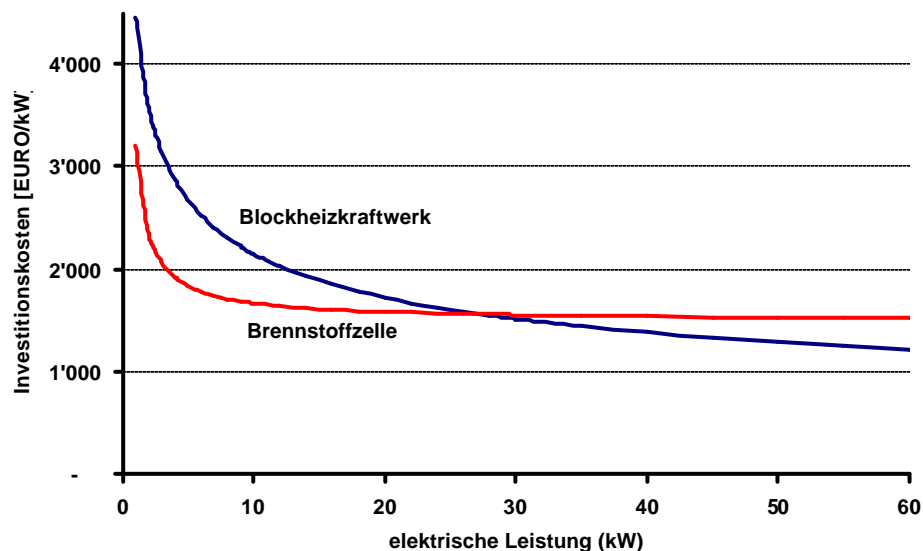
Spezifische Investitionskosten von Brennstoffzellen-Systemen und Blockheizkraftwerken 5
