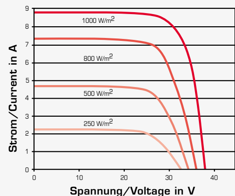
Beispiel AC-250M/156-60S
